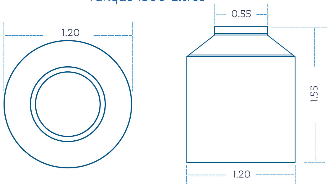
Tanque 1500 Litros
